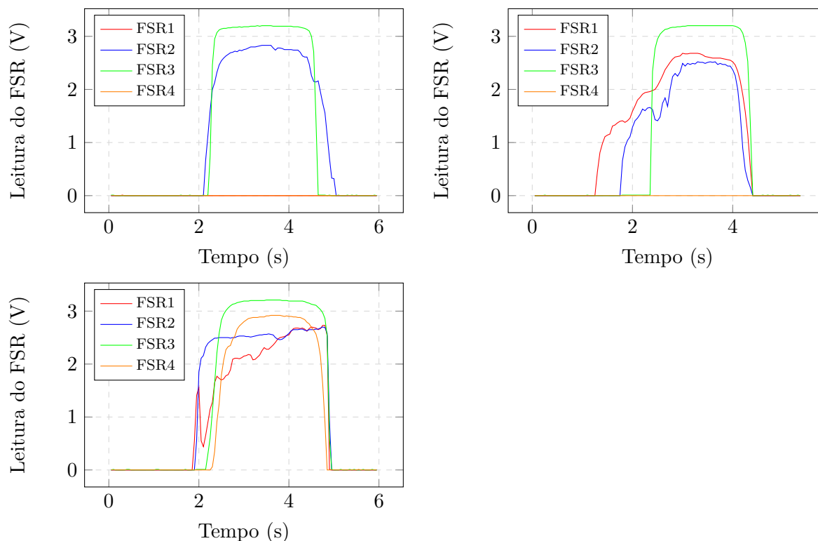
Figura 4.28: Gráfico da tensão de saída dos sensores durante a aplicação de força sobre 2, 3 e 4 sensores em simultâneo.
